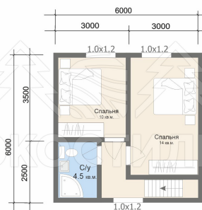
План 2 этажа
