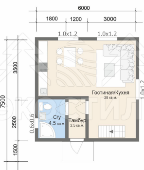
План 1 этажа
